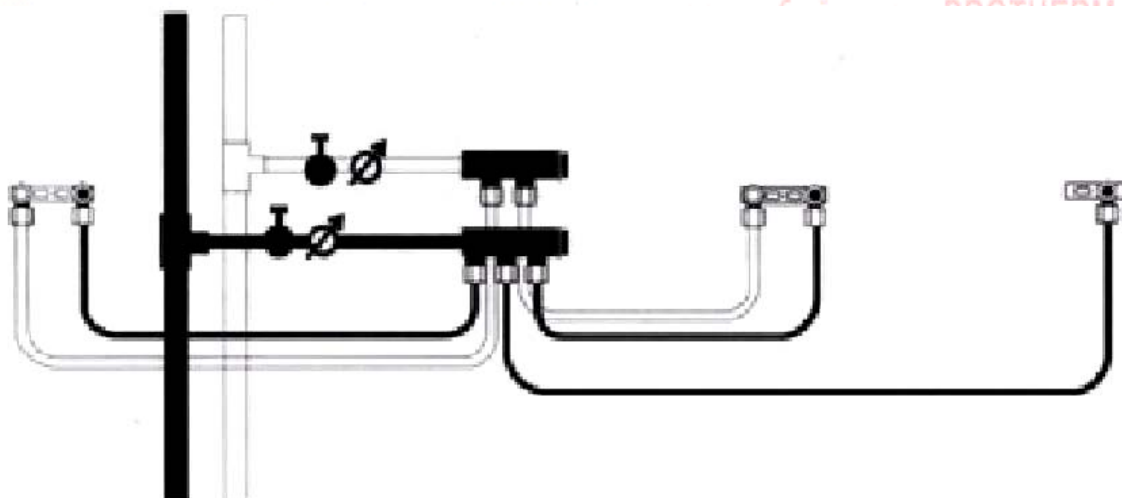
Рис 1. Коллекторная схема
